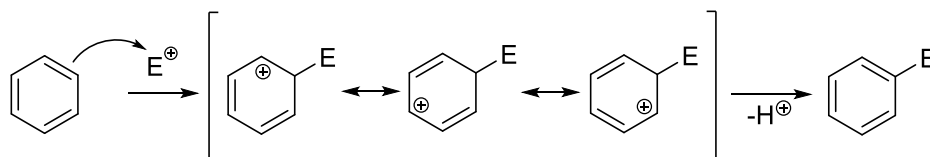
Schema 1: Allgemeiner Mechanismus der elektrophilen aromatischen Substitution, E = Elektrophil.
