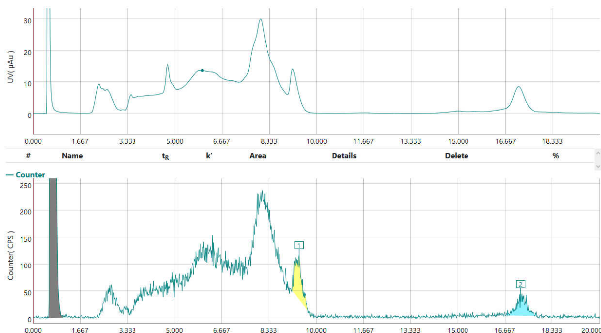
Abbildung 10: HPLC-Chromatogramm (oben: UV-Absorption, unten: Zählrate) der Dakin Reaktion (Tabelle 8, Reaktion 8); grau: Referenzpeak, gelb: 2-[ 18 F]Fluorbenzoesäure ([ 18 F] 12 ), blau: 2-[ 18 F]Fluorbenzaldehyd ([ 18 F] 11 ), kein 2-[ 18 F]Fluorphenol ([ 18 F] 13 ), viele Nebenprodukte; Reaktionsbedingungen: ~4,22 μl (40 mmol, 1Äq.) 2-[ 18 F]Fluorbenzaldehyd ([ 18 F] 11 ), 50 μl (490 mmol, 12 Äq.) H 2 O 2 , 26,7 μl 30%-ige NaOH in Methanol, HPLC-Bedingungen: 30 % wässriges Acetonitril + 0,2 Vol% Essigsäure, 80°C, 20 μl Probenvolumen, Gemini 5 μm C18 Säule, Fließgeschwindigkeit 1 ml/min.
