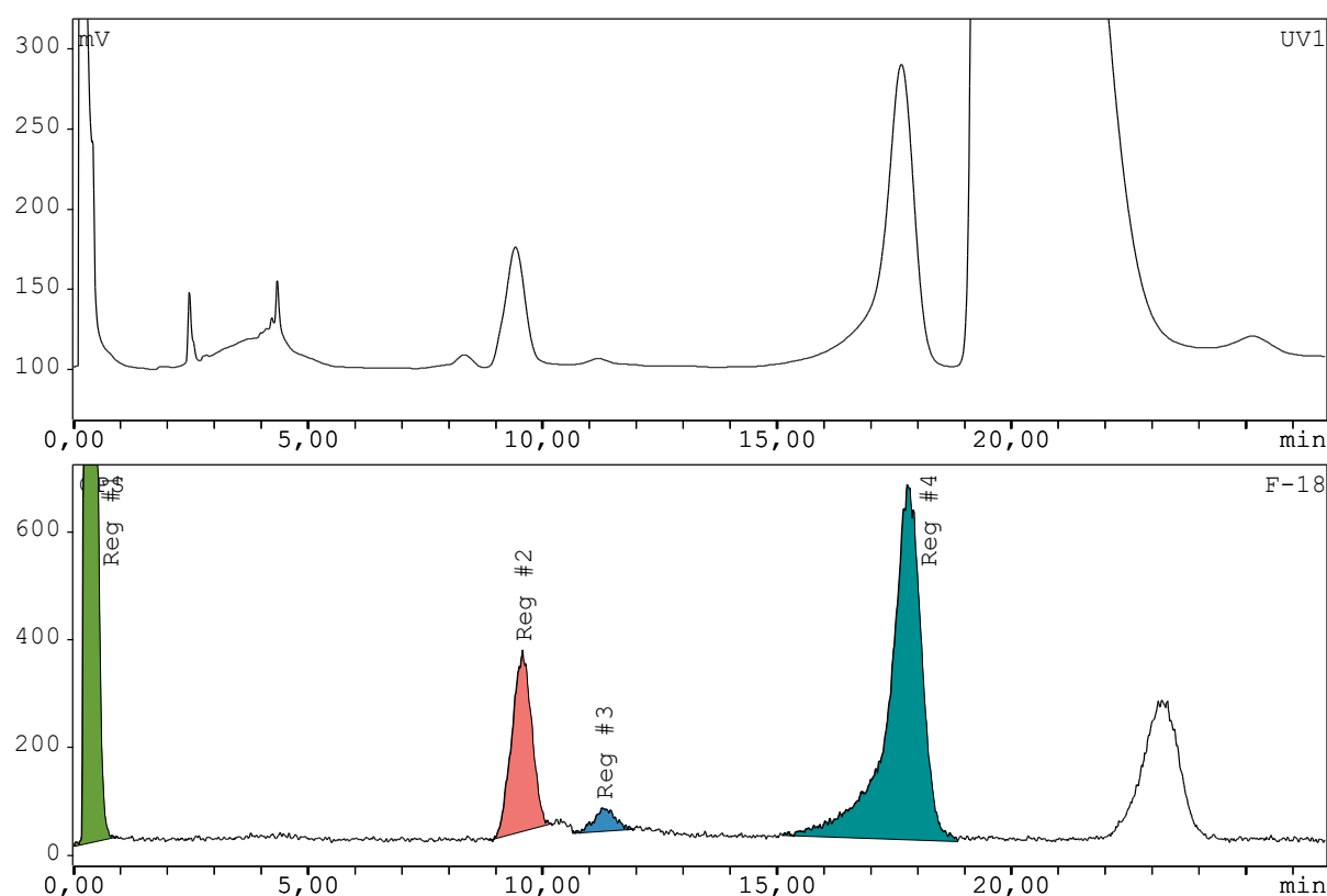
Abbildung 7: HPLC-Chromatogramm (oben: UV-Absorption, unten: Zählrate) der BVO von 2-[ ^{18}\text{F} ]Fluorbenzaldehyd mit mCPBA und Phosphorsäure; grün: Referenzpeak, rot: 2-[ ^{18}\text{F} ]Fluorbenzoesäure ([ ^{18}\text{F} ]12), blau 2-[ ^{18}\text{F} ]Fluorphenol ([ ^{18}\text{F} ]13), türkis: 2-[ ^{18}\text{F} ]Fluorbenzaldehyd ([ ^{18}\text{F} ]11); Reaktionsbedingungen: \sim 4,22 \mu\text{l} (40 mmol, 1Äq.) 2-[ ^{18}\text{F} ]Fluorbenzaldehyd ([ ^{18}\text{F} ]11), 51,1 mg (240 mmol, 6Äq.) mCPBA, 15 \mu\text{l} konz. Phosphorsäure in
