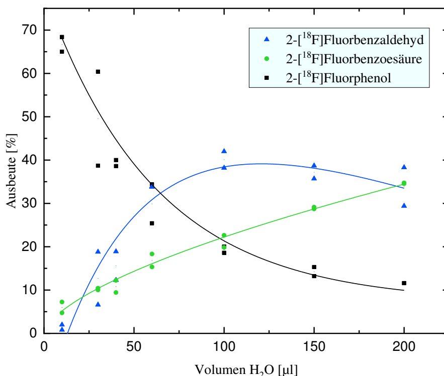
Abbildung 6: Diagramm der Ausbeuten der Versuche der BVO mit m CPBA als Oxidationsmittel und Schwefelsäure als Katalysator in Trifluorethanol mit unterschiedlichen Mengen zugesetztem Wasser bei 80°C; n =2; radiochemische Ausbeuten mittels HPLC bestimmt: nach 30 min BVO.
